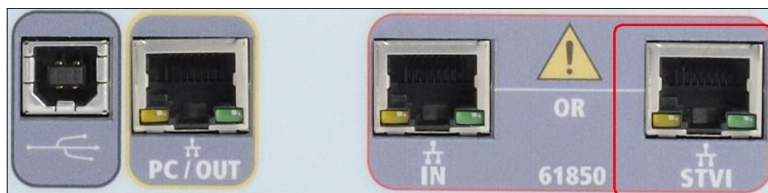
Figura 3 Puerto STVI en MRCT
