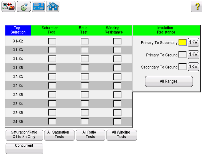
Figura 24 Ejecutar todas las pruebas - Configuración
