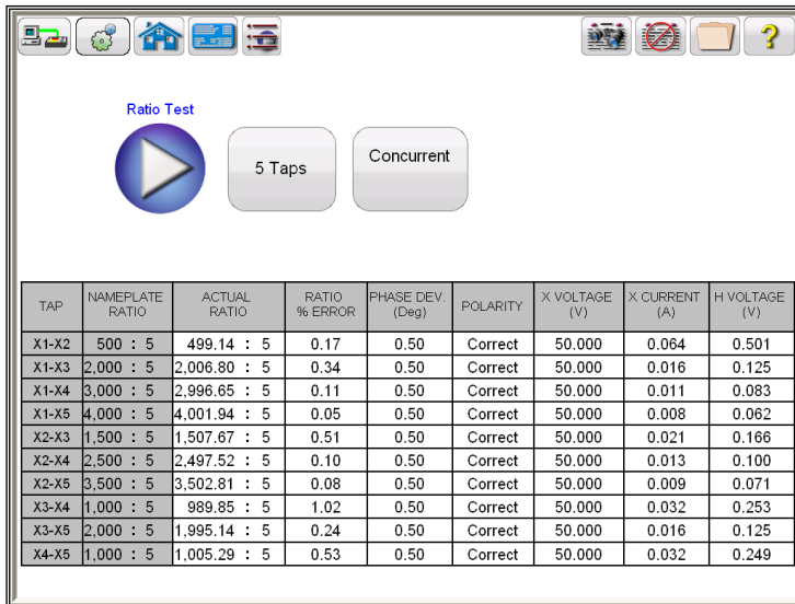
Figura 39 Resultados de la Prueba de Relación – Simultáneo
