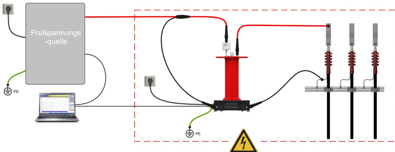
Verbotzone und Prüfbereich nach DIN EN 50191 (VDE 0104)
