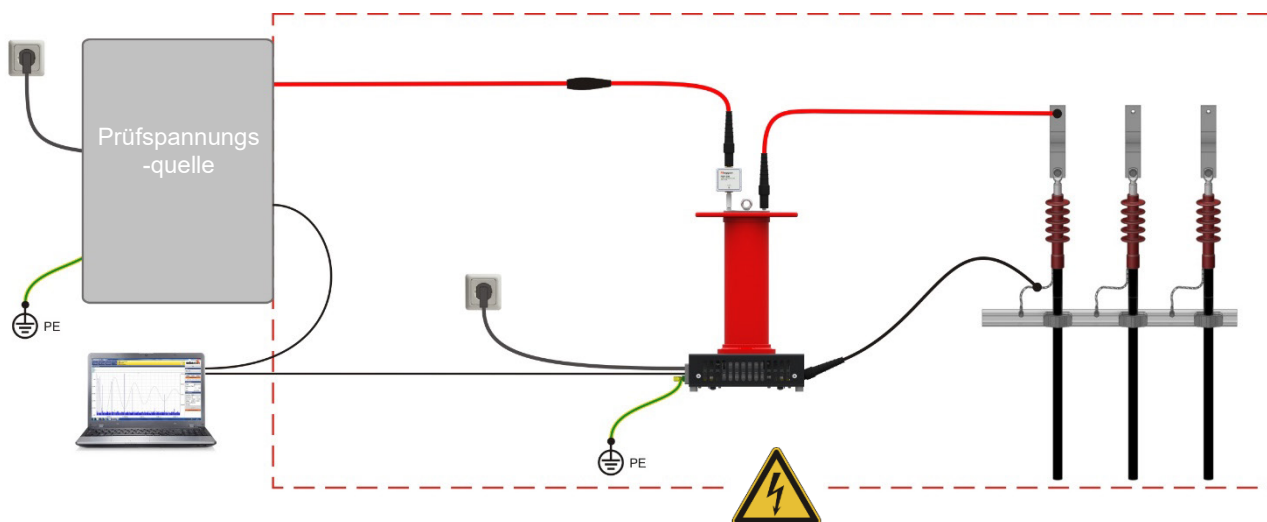
Verbotzone und Prüfbereich nach DIN EN 50191 (VDE 0104)
