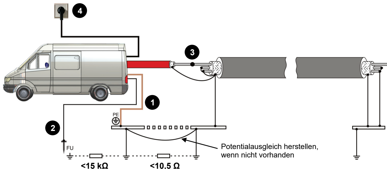
Bild 6: Elektrischer Anschluss des VLF Test Systems
