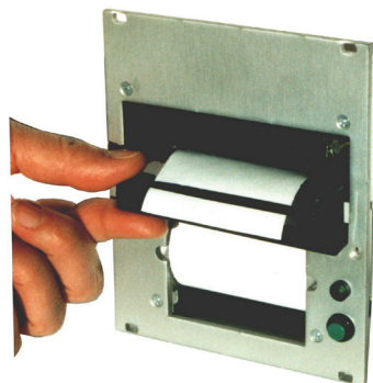
Bild 41: Farbbandkassette einlegen
