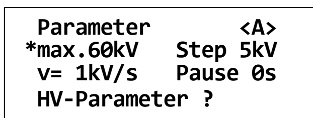
Bild 19: Setup, Parameter
