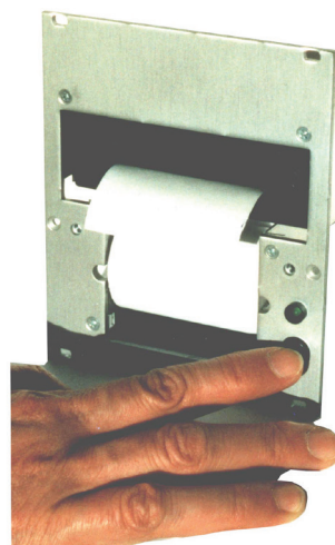
Bild 43: Papiervorschubtaste
