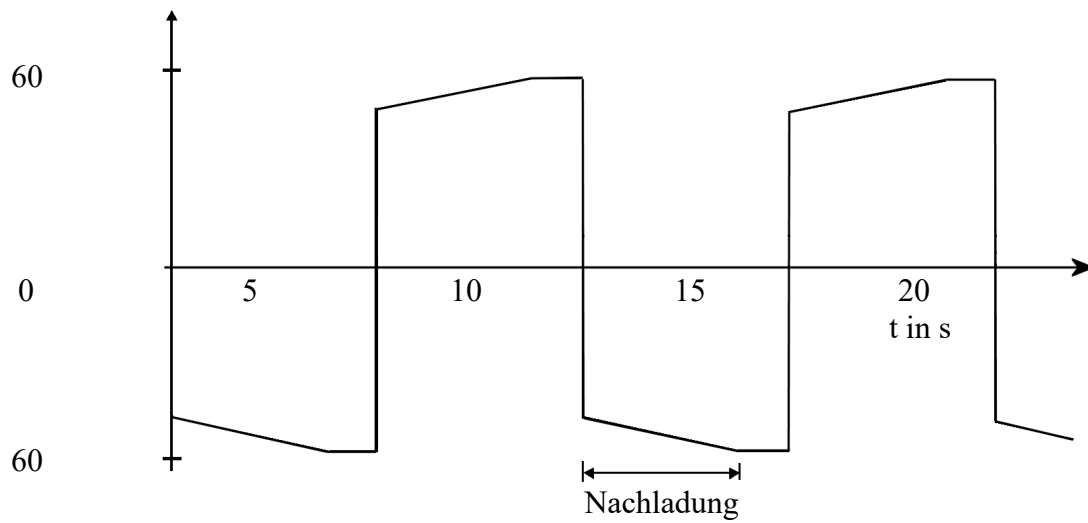
Bild 1: Darstellung Prüfspannungsverlauf
