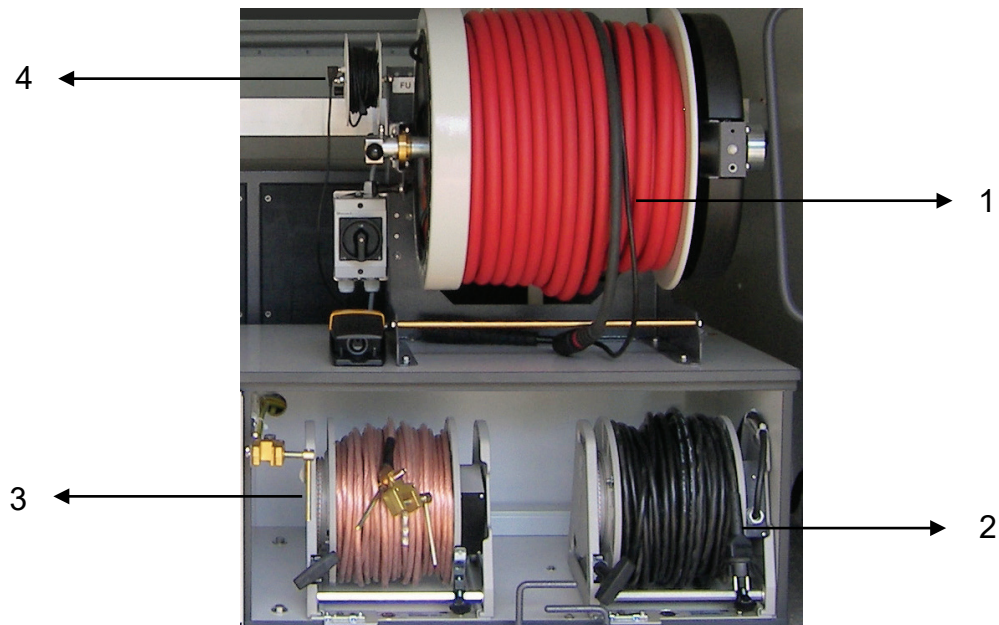
Bild 7: Anschlussequipment
