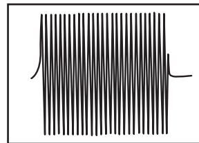
Figura 5. Con red de compensación de impedancia, un reconector con una bobina de 50 amperios y una corriente de prueba inicial de 210 amperios en funcionamiento en 0,783 segundos sin disminución de corriente significativa. El resultado estaba dentro de las especificaciones del fabricante.
