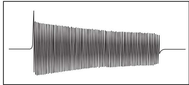
Figura 4. Sin red de compensación de impedancia, un reconector con una bobina de 50 amperios y una corriente de prueba inicial de 210 amperios en funcionamiento 2,641 segundos (tres veces las especificaciones del fabricante).
