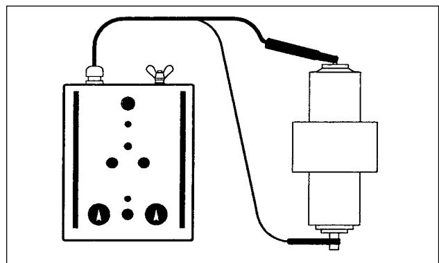
Diagrama de conexiones para la VIDAR
