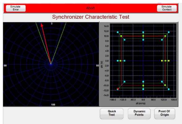
Opcja dynamicznych punktów pomiarowych w teście synchronizmu
