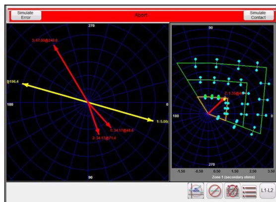
Ekran pomiarowy prezentujący w czasie rzeczywistym przebieg testu zabezpieczenia o charakterystyce poligonalnej (QUAD)
