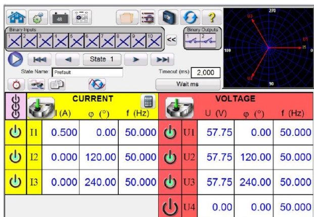
Ekran testów sekwencyjnych
