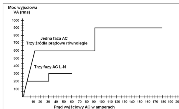
Charakterystyka mocy źródeł prądowych FREJA 546
