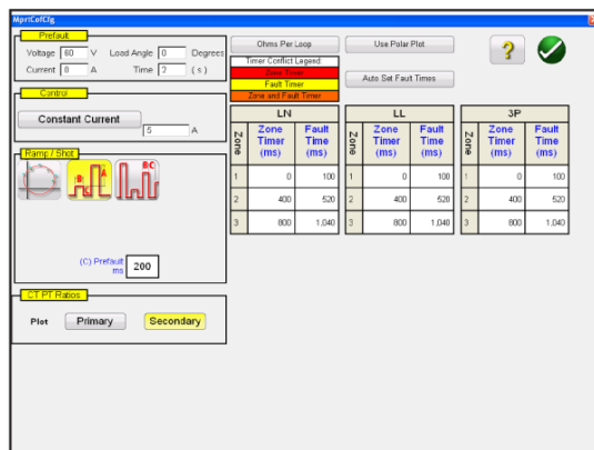
Ekran konfiguracji testu opartego na rodzajowej charakterystyce poligonalnej
