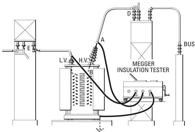
Figura 33: Conexiones para probar la resistencia del aislamiento de bushings y devanados de alta tensión de un transformador y el interruptor de desconexión de alta tensión en paralelo con referencia a tierra, pero sin verse afectados por las fugas entre los devanados de alta y baja tensión mediante el uso de la conexión de la protección.
