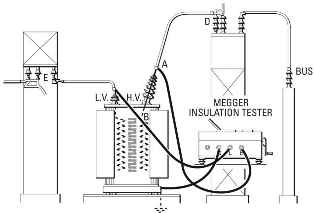
Figura 34: Conexiones para probar la resistencia del aislamiento entre los devanados de alta y baja tensión, sin verse afectados por la fuga a tierra.
