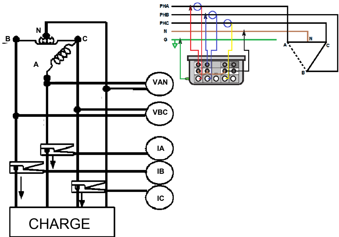
Méthode de mesure à 2½ wattmètres à 4 fils Red-Leg ouverts
