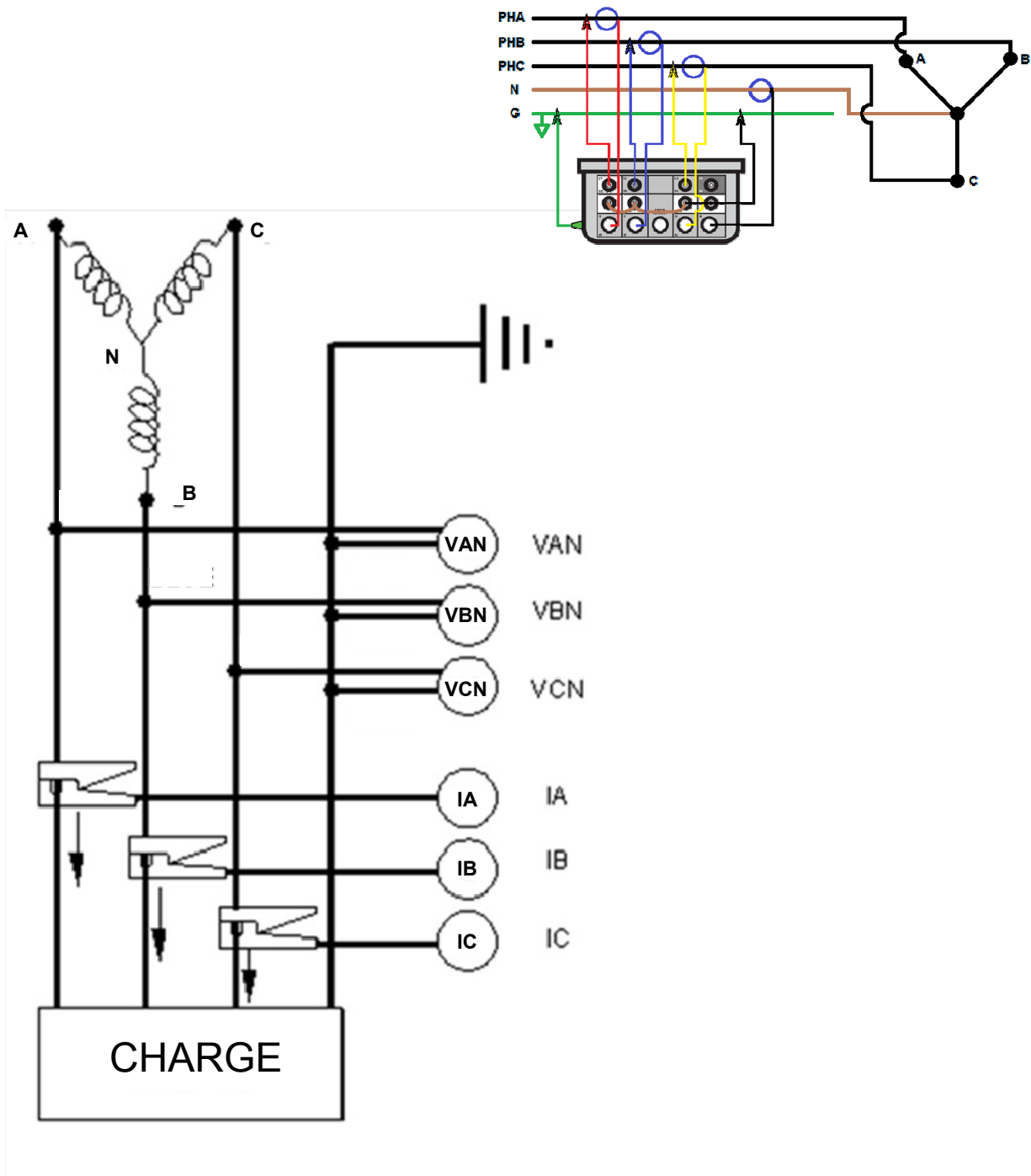
Connexion en étoile flottante Méthode de mesure à 3 wattmètres à 4 fils raccordés en étoile
