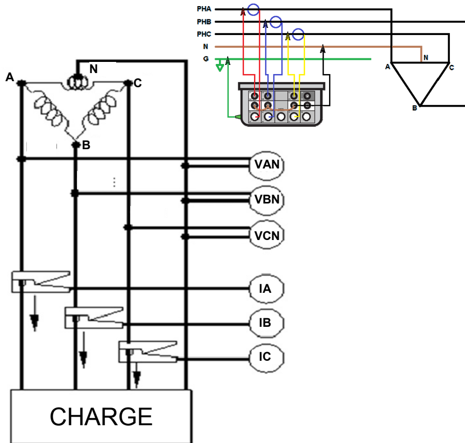
Méthode de mesure à 3 wattmètres à fils en triangle
