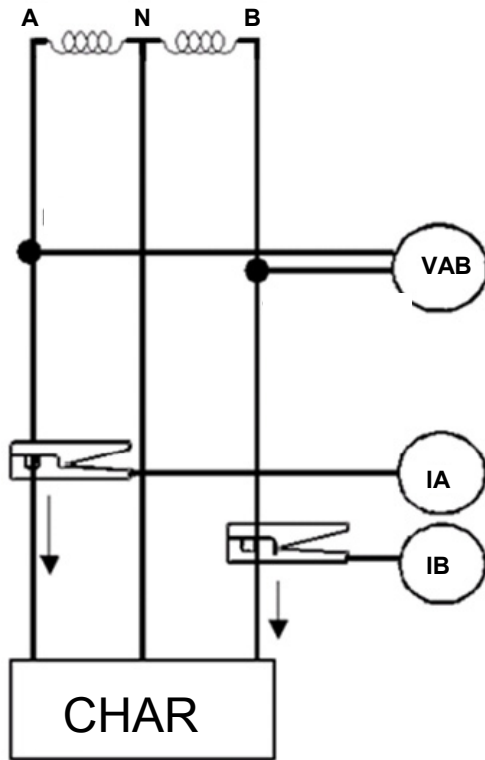
Appareil de mesure résidentiel trifilaire monophasé
