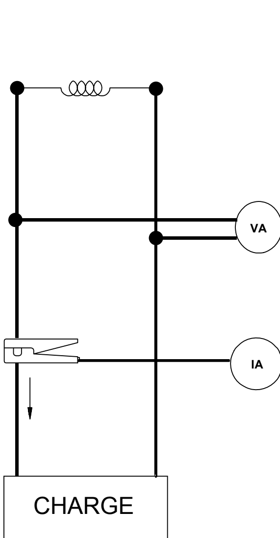
Un seul wattmètre bifilaire monophasé
