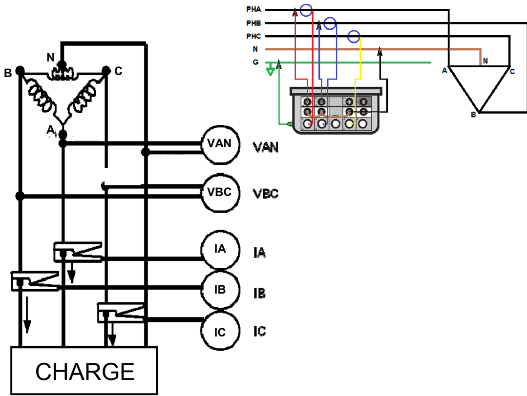
Méthode mesure à 2½ wattmètres à 4 fils en triangle Gred-Leg
