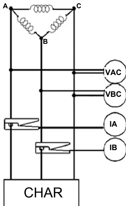
Méthode de mesure à 2 wattmètres trifilaires raccordés en triangle
