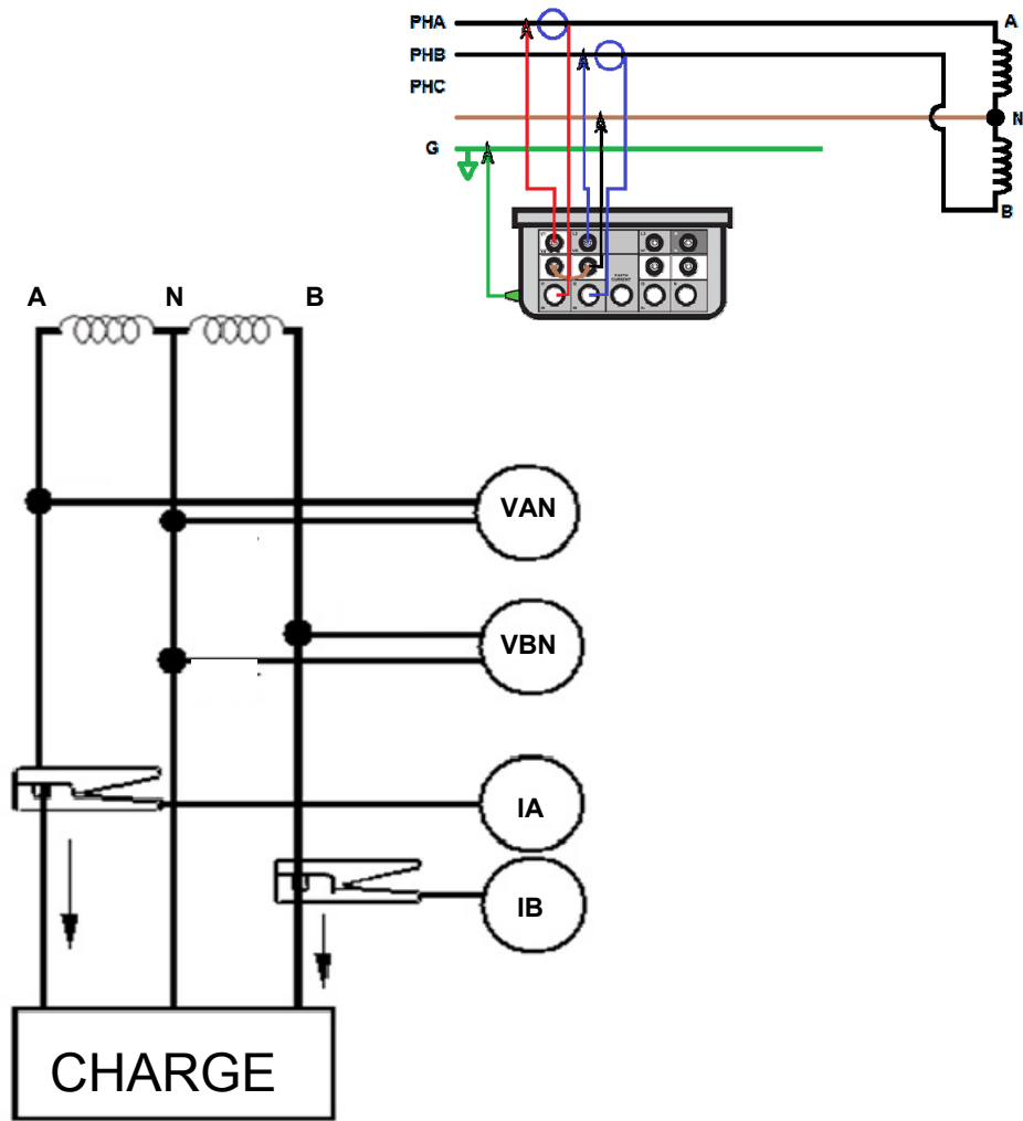
Appareil de mesure de réseau trifilaire
