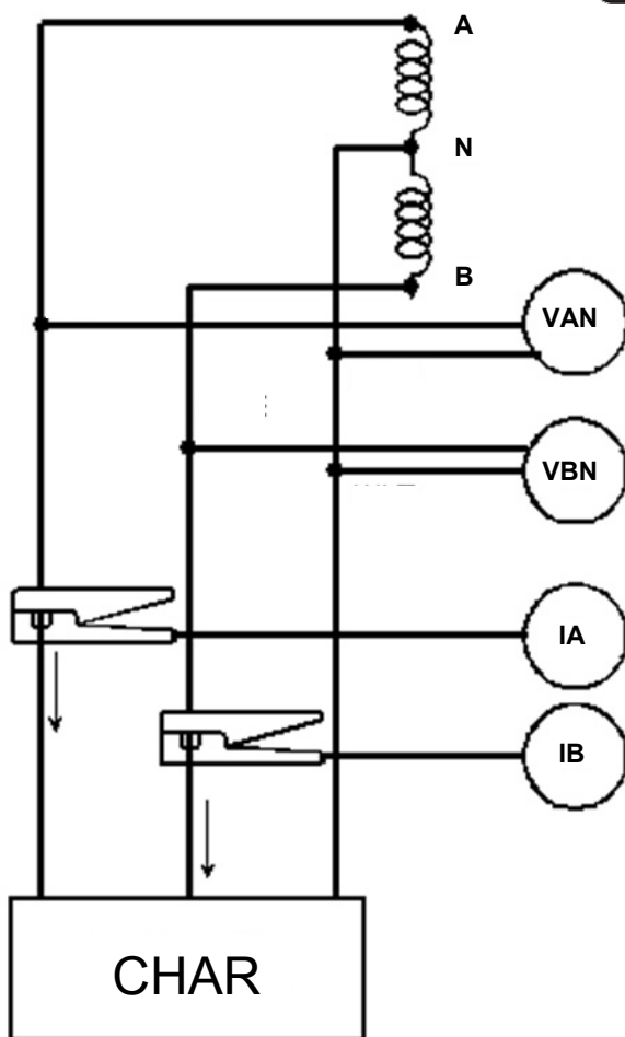
Méthode de mesure à 2 wattmètres trifilaires de phase auxiliaire
