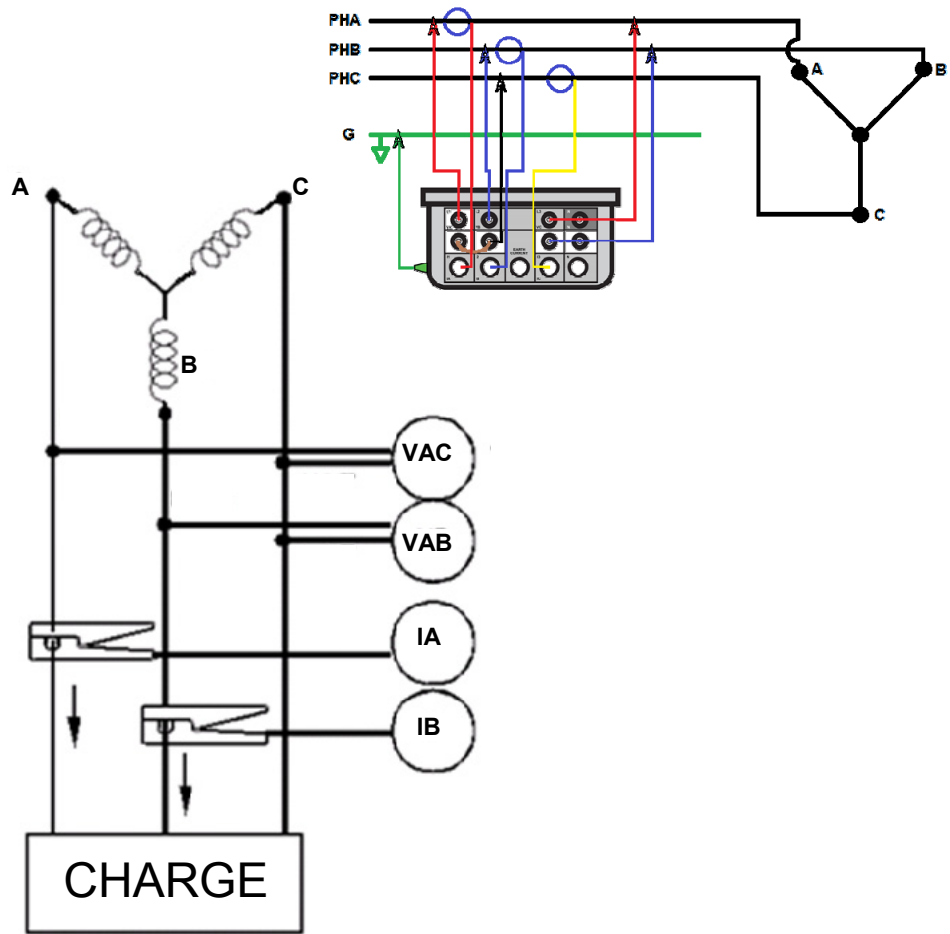
Méthode de mesure à 2 wattmètres trifilaires raccordés en étoile
